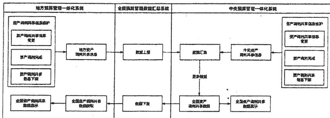
图 3: 资产调剂共享信息发布流程
