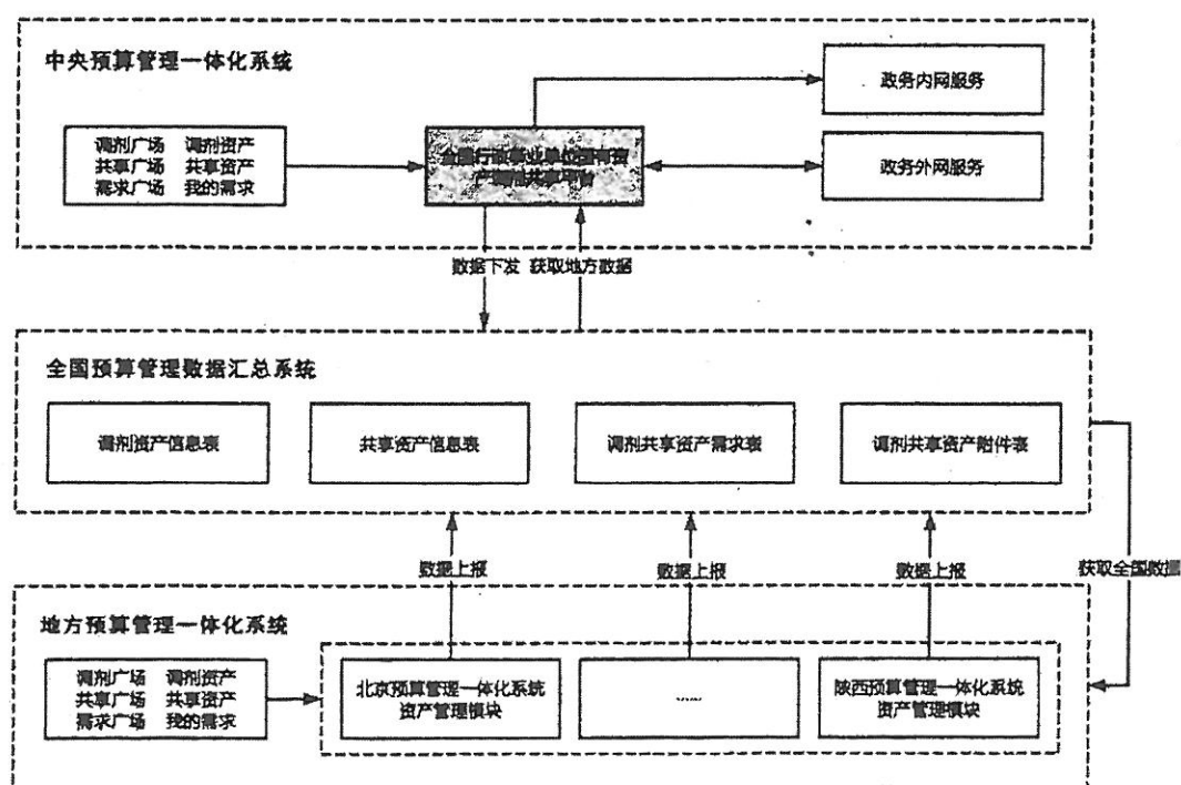
图 1：平台功能框架
