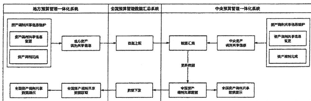
图 4：资产调剂共享信息更新流程
